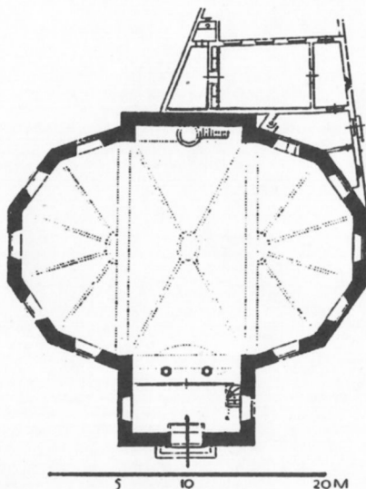
PLATTEGROND KERK
